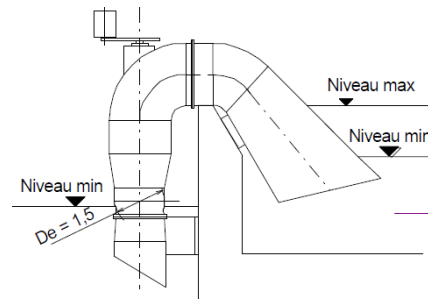
Axiale, siphon 1.0 - 3.5 m
