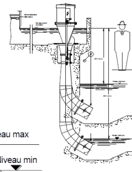
Axiale, Pico turbine 1 - 5 m
